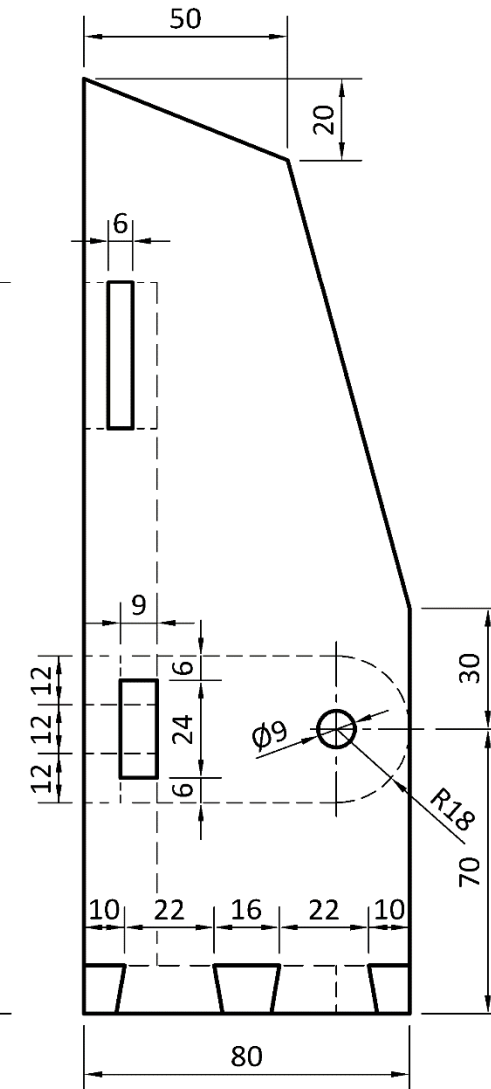
End View/Taobhchló
