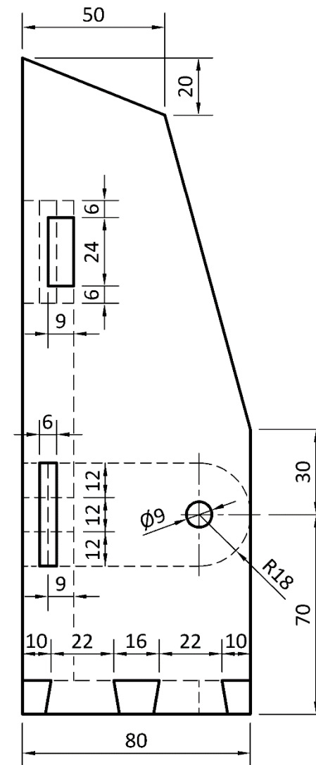
End View/Taobhchló
